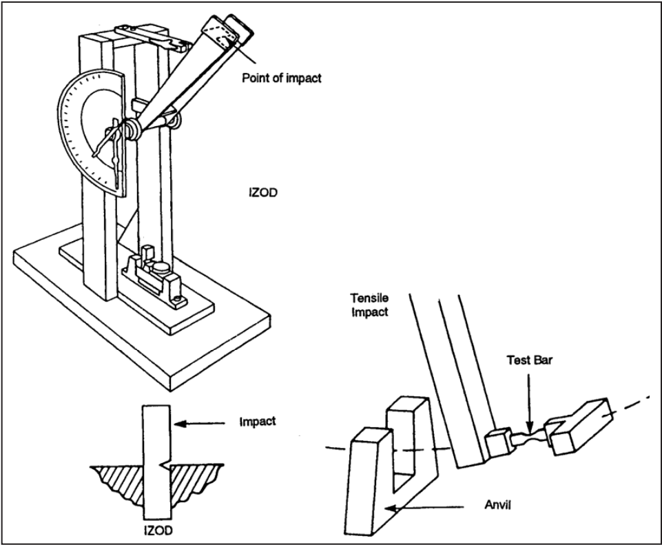
Figure 14 Izod Test
